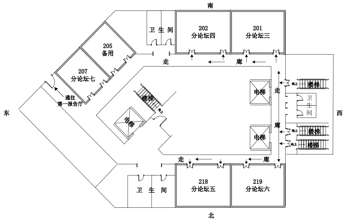
逸夫楼二层平面示意图
